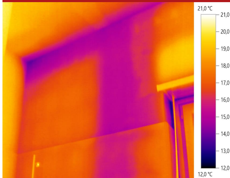
Figura 4: Parete perimetrale non isolata
