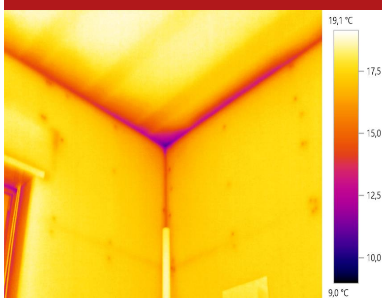
Figura 6: Parete perimetrale isolata
