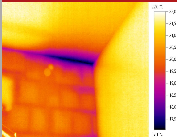
Figura 3: Parete perimetrale non isolata
