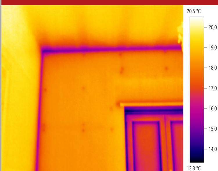
Figura 5: Parete perimetrale isolata
